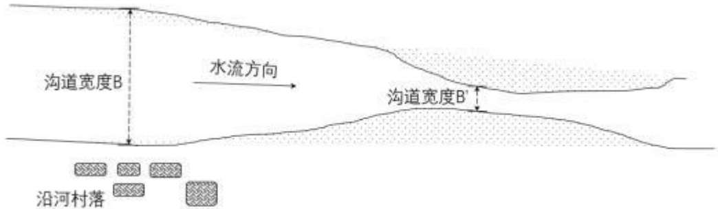
图 0-20 下游沟道束窄大水致灾示意图
